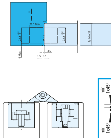
Sección puerta enrasada
