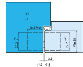
Sección puerta enrasada y solapada
